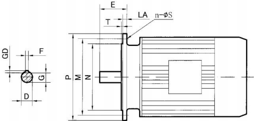
常用电机参数（IEC标准电机尺寸）
